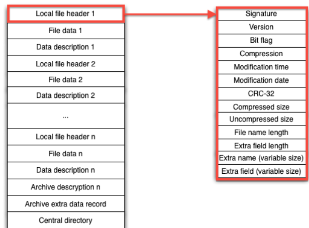
Structure d'une archive ZIP
