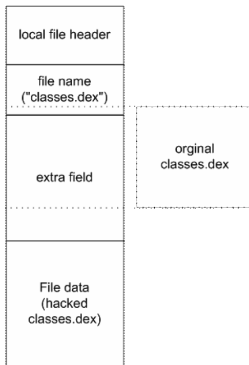
Schéma d'exploitation de vulnérabilité « extra_field »
